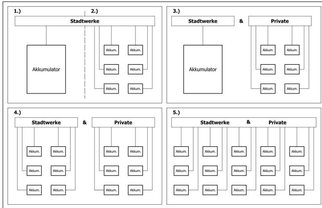
Abb. 1: Varianten für zentrale Groß- und dezentrale Klein-Akkumulatorenspeichersysteme für Stadtwerke (Eigene Darstellung)
