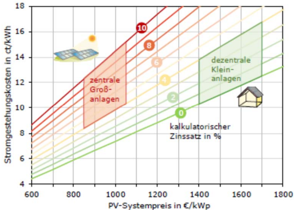
Abb. 3: Stromgestehungskosten für netzgekoppelte PV-Systeme sowie die Bereiche typischer Systempreise und Renditeerwartungen für dezentrale und zentrale Systeme (Annahmen: jährliche Betriebskosten 2 % der Investitionskosten, spezifischer Ertrag 950 kWh/kWp; Quelle: Weniger et al. 2015).
